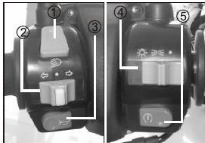
Schaltereinheiten links und rechts
